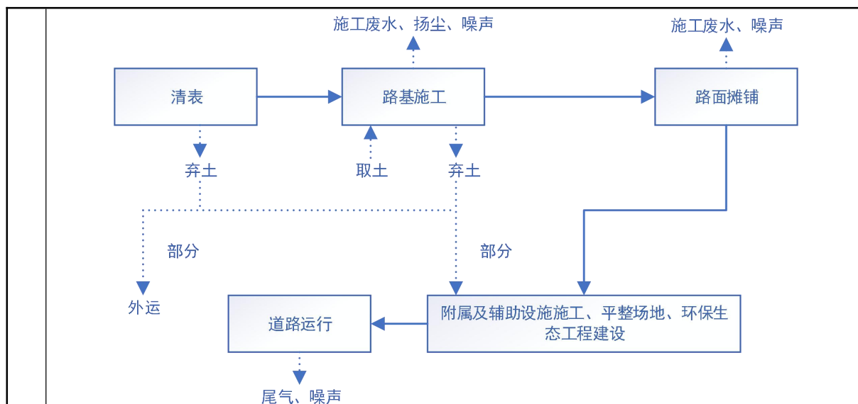
图 2-1 施工期工艺及污染物产排流程图
