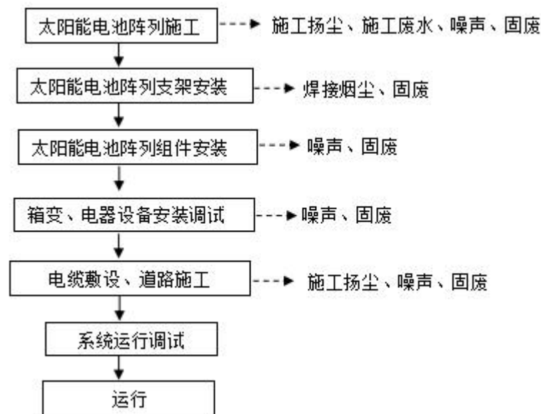
图 2-2 施工工艺流程图
