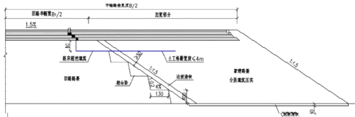
图 2-3 路基横向拼宽设计图
