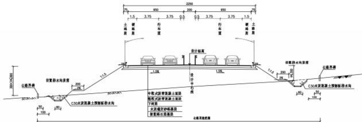
图 2-2 一级公路整体式 22.5m 路基标准横断面（K4+200-K10+264.54）
