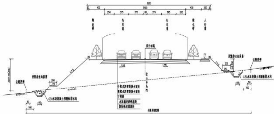
图 2-1 一级公路整体式 32.0m 路基标准横断面（K0+000-K4+200）
