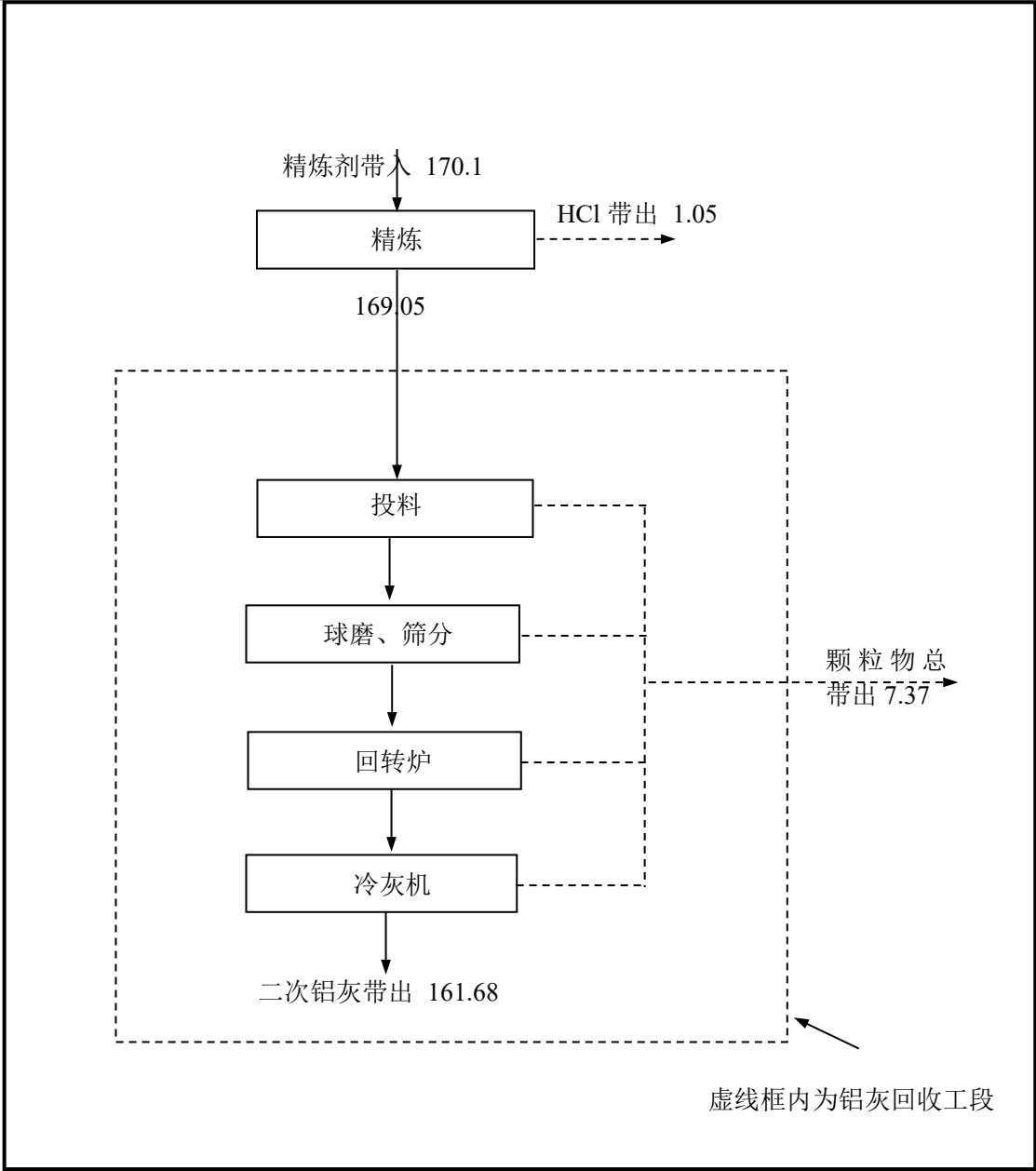
图 3.2-5 本项目氯物料平衡图 t/a
