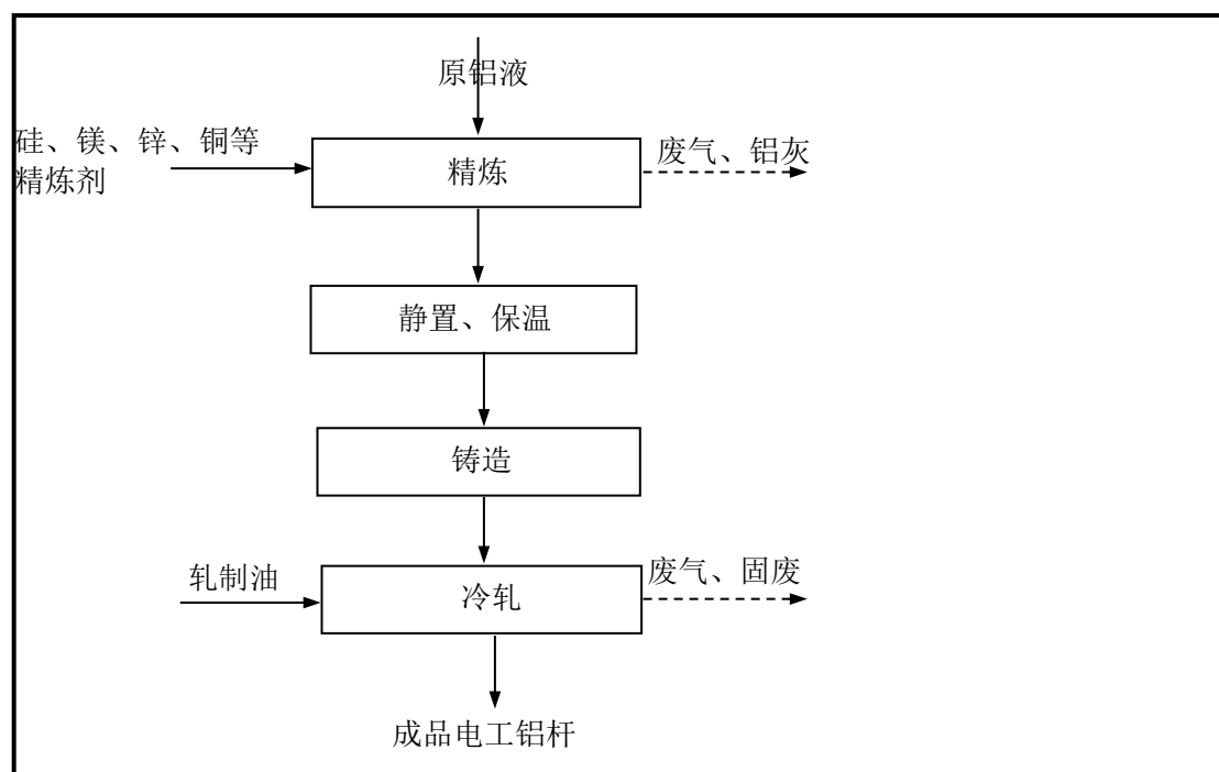
图 3.2-2 本项目电工铝杆生产工艺及产污环节图
