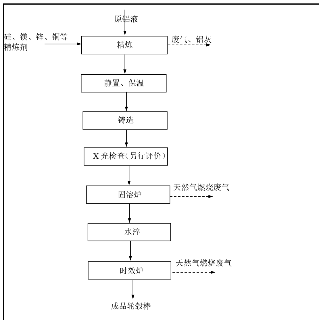
图 3.2-3 本项目轮毂棒生产工艺及产污环节图
