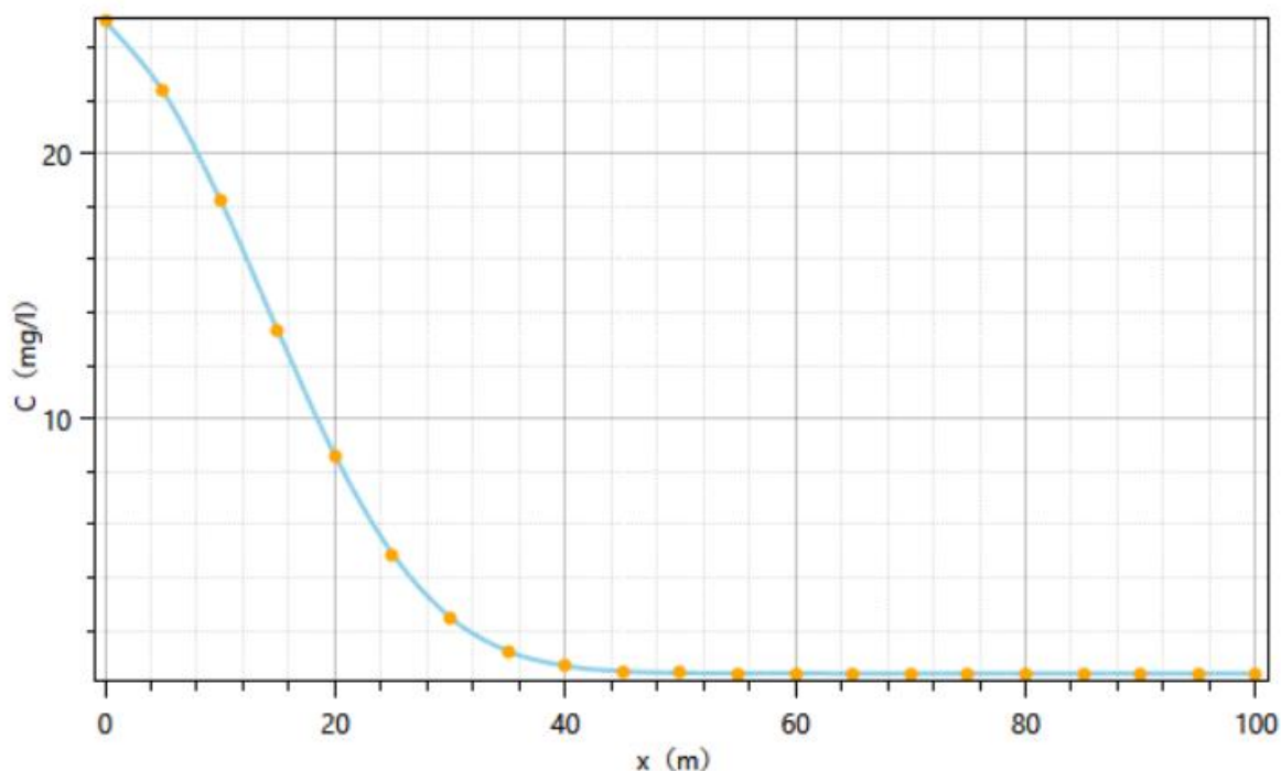
图 5.2-11 氨氮 7300d 运移情况示意图
