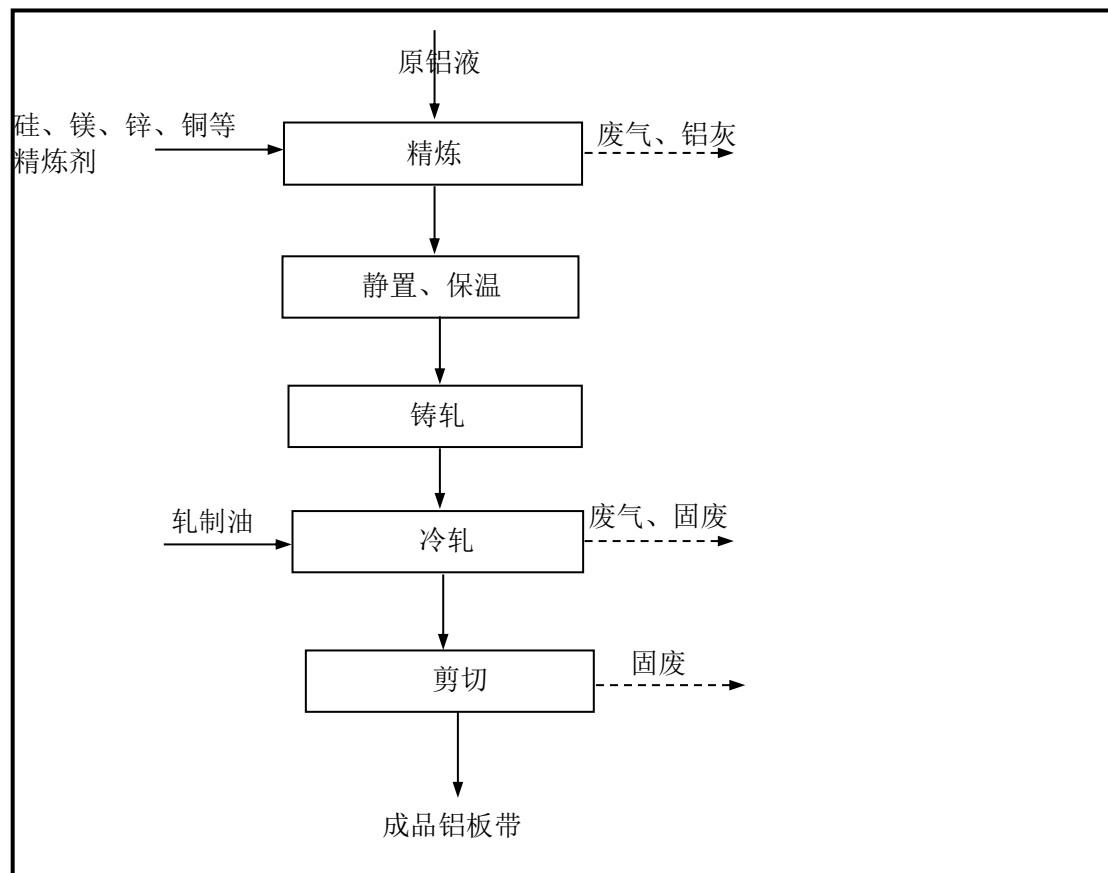
图 3.2-1 本项目铝板带生产工艺及产污环节图
