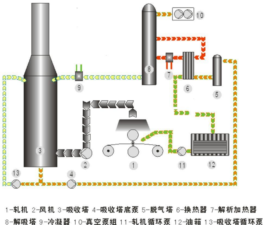
图 6.2-2 全油回收油雾净化装置结构图
