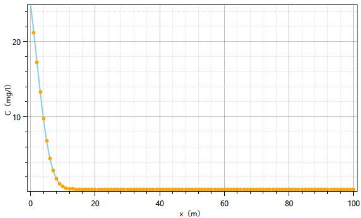
图 5.2-10 氨氮 100d 运移情况示意图
