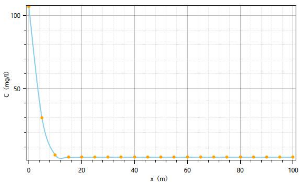
图5.2-8 耗氧量100d运移情况示意图
