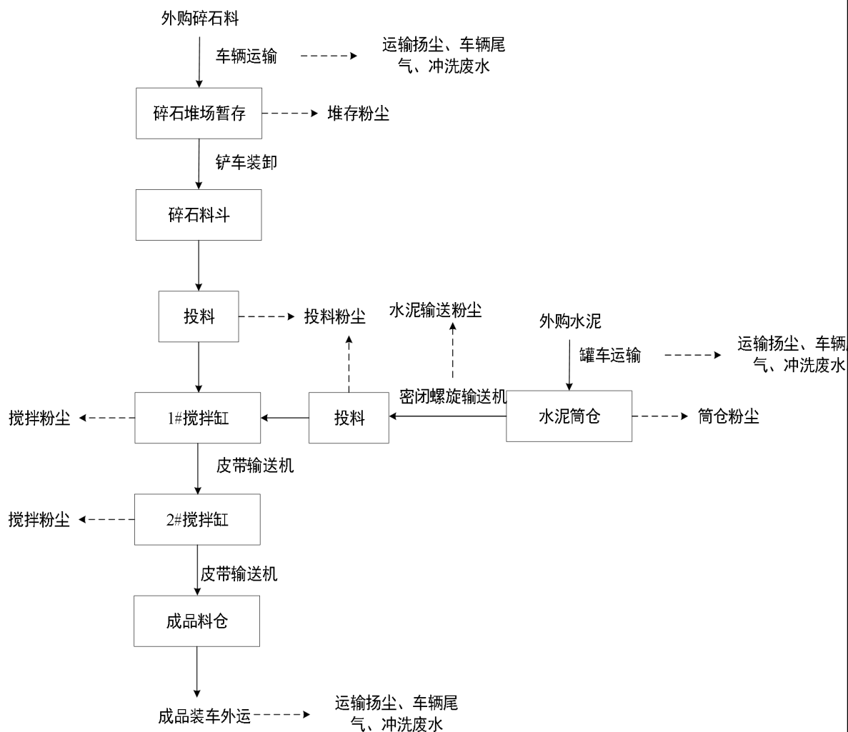
图 2-2 运营期水稳站工艺流程及产污节点图
