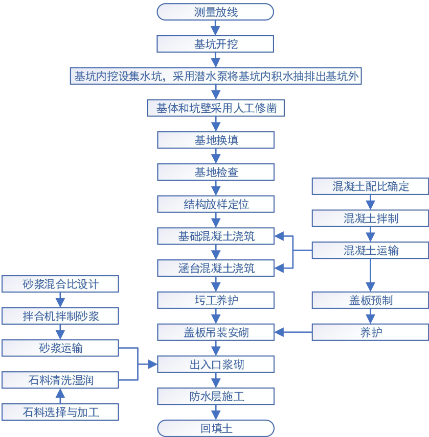
图 2-3 桥涵施工期工艺
