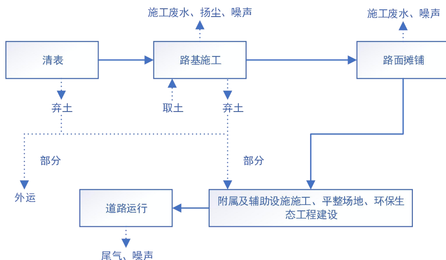
图 2-2 施工期工艺及污染物产排流程图
