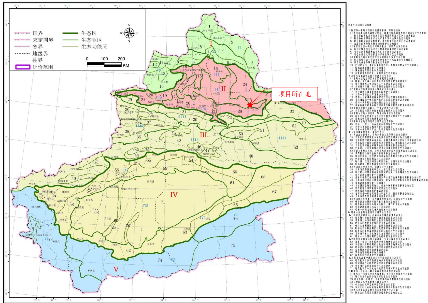
附图 9: 生态功能区划图
