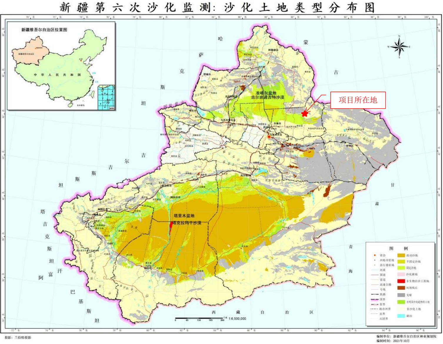
附图 12：新疆第六次沙化监测沙化土地分布图
