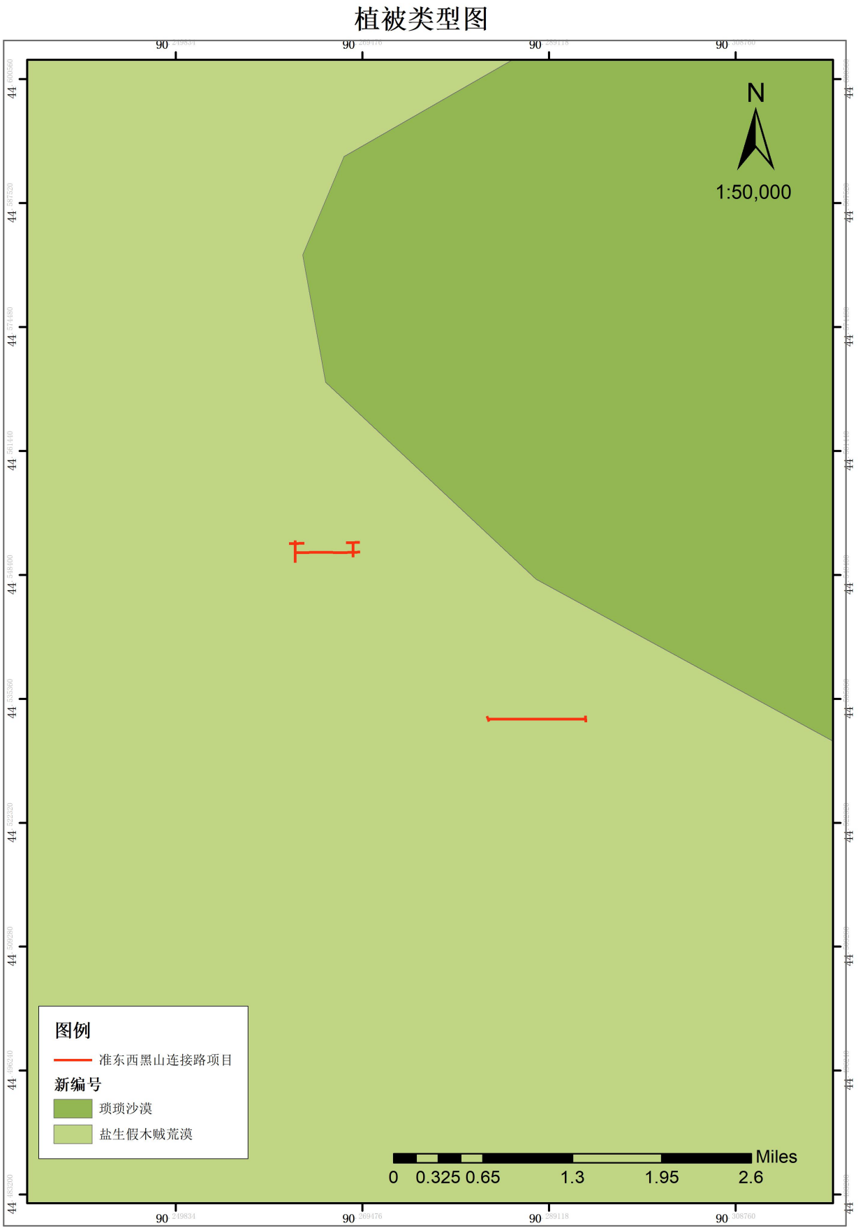
附图 12: 植被类型图
