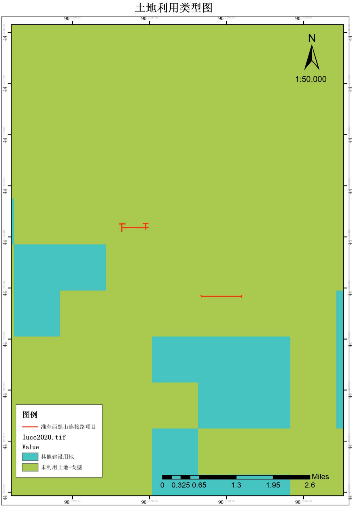
附图 10：土地利用图
