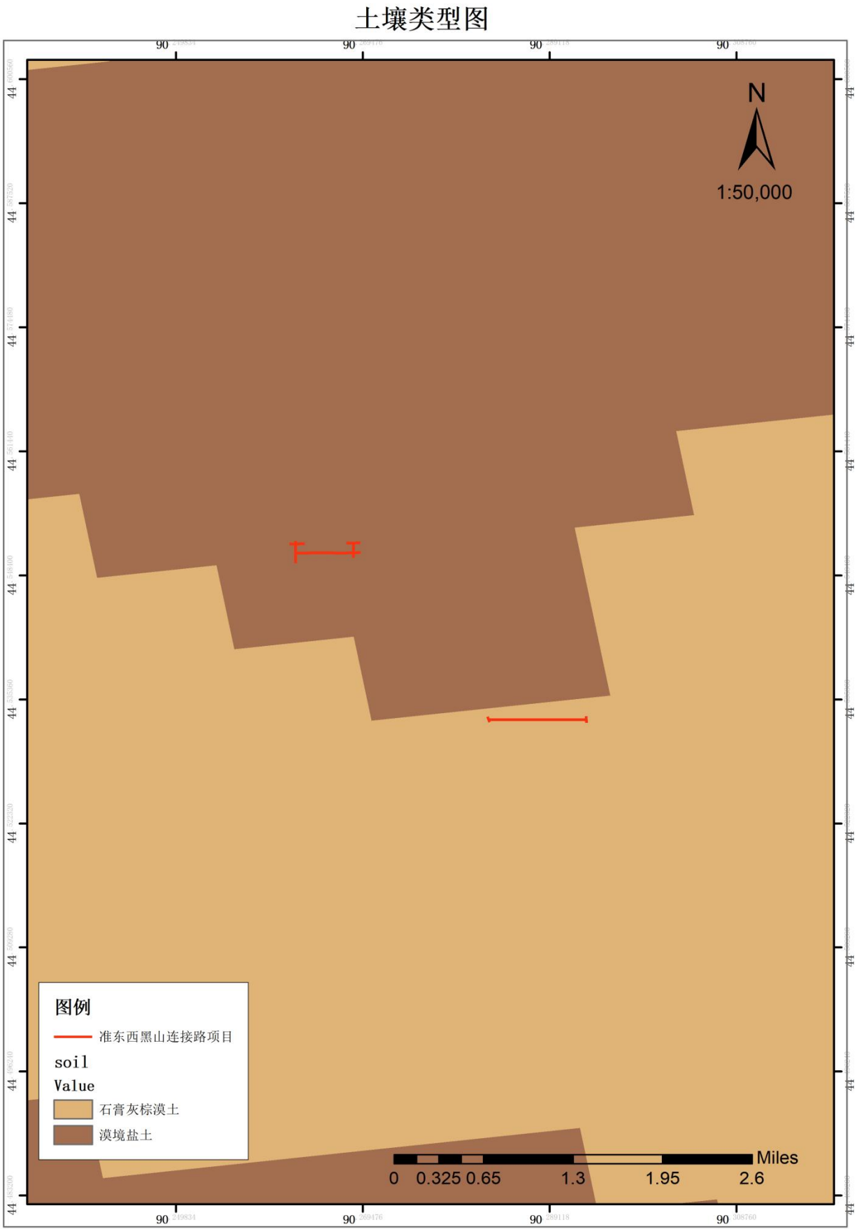
附图 11：土壤类型图
