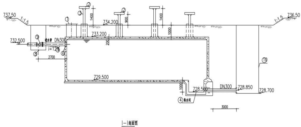
图3.2-3垃圾填埋场剖面结构示意图
