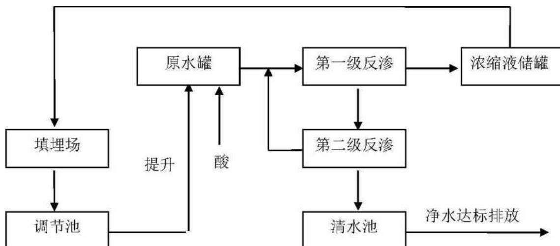
图7.2-2 渗滤液处理工艺流程示意图
