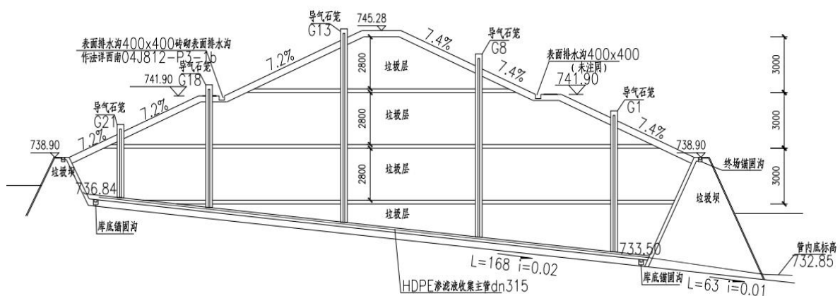
图3.2-5 填埋场封场结构图
