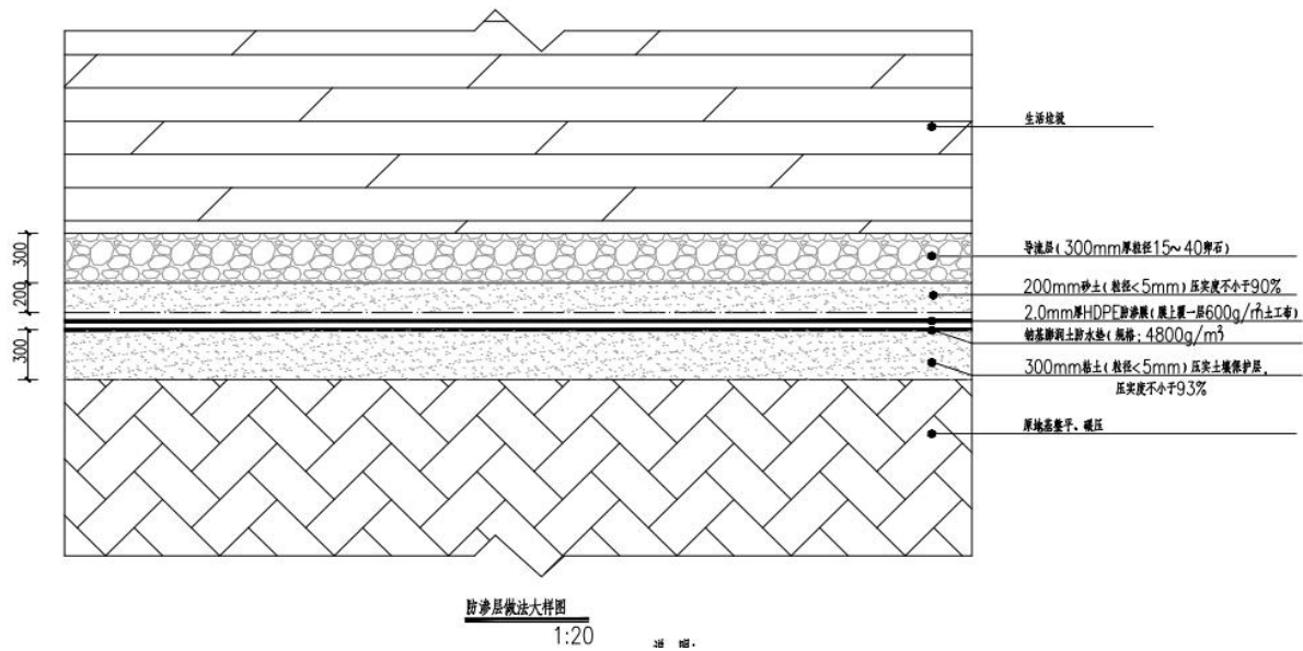
图3.2-2库底、侧壁、垃圾坝防渗层结构图
