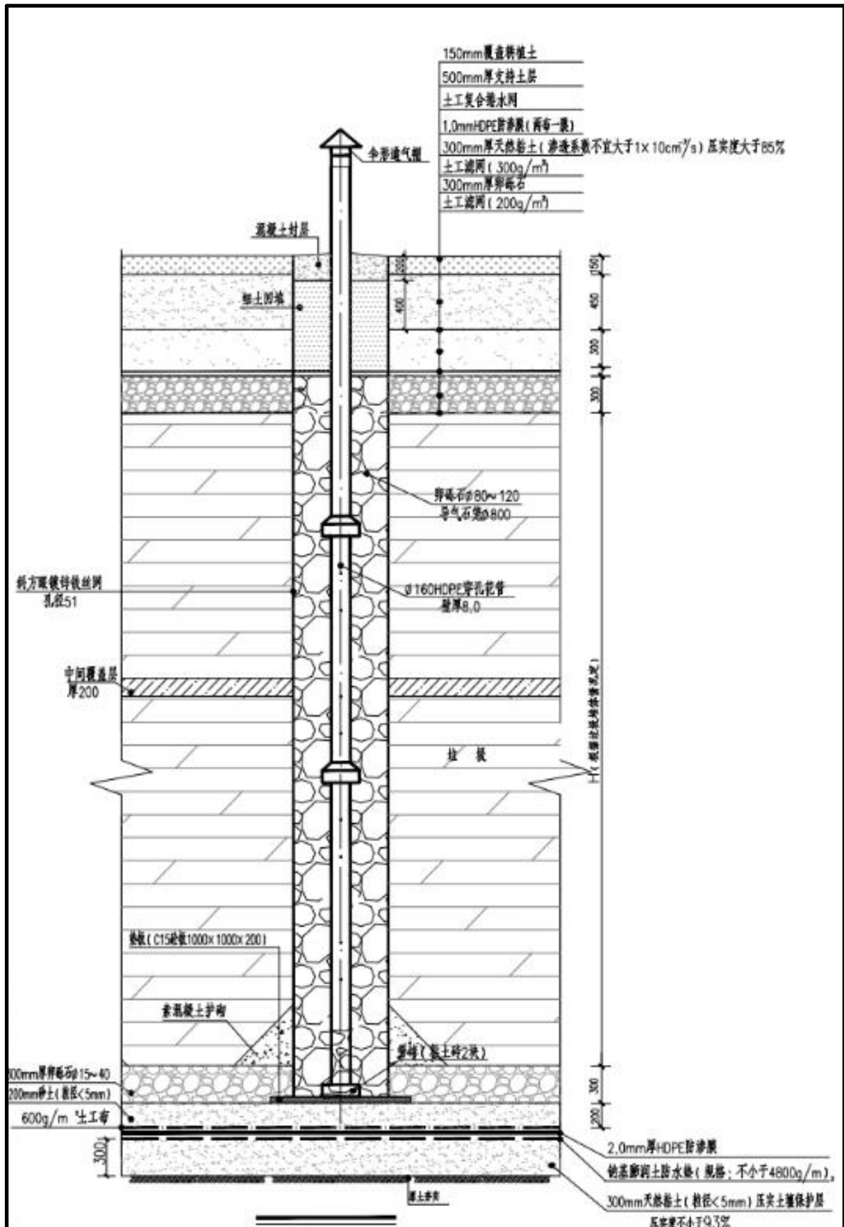
图3.2-4填埋场封场结构图
