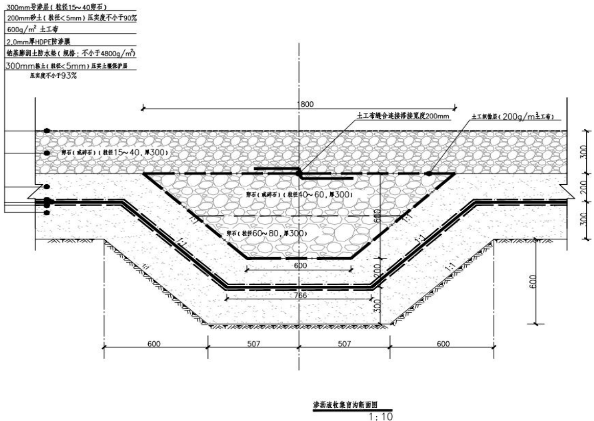
图3.2-4 渗沥液收集盲沟断面图
